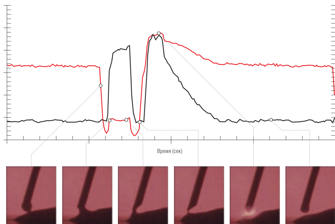
Механика процесса сварки металлическим электродом в инертном газе с системой уменьшения налипания брызг (SRS)
