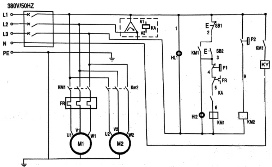
Рис.6.3.2 Модели CRD 14-18-22-28
