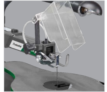
Abblasvorrichtung entfernt groben Sägestaub aus dem Schnittbereich
