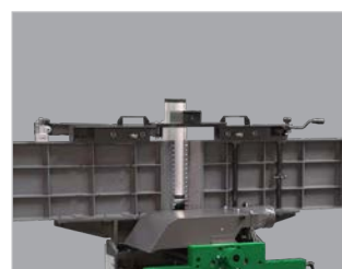
ADH 31-4 C Gerüstet zum Dickenhobeln
