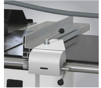
Großer Aluminium-Parallelanschlag auf Rundstangenführung mit Feineinstellung
